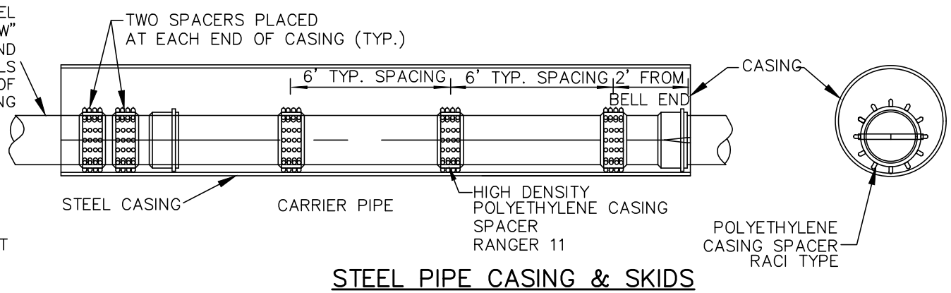
STEEL PIPE CASING & SKIDS N.T.S.
