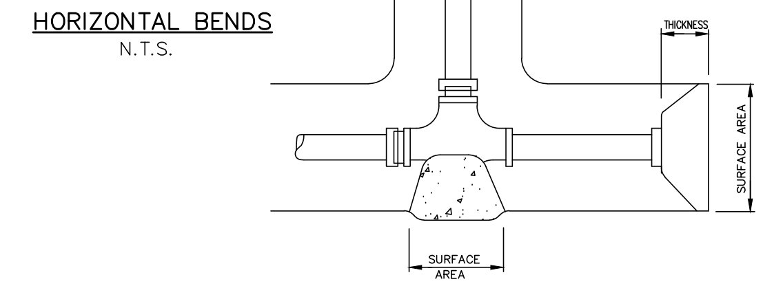
TEES & DEAD ENDS N.T.S.
