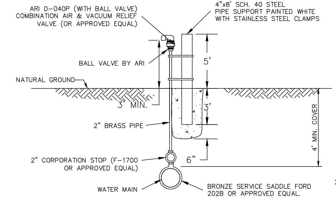
AIR RELEASE VALVE N.T.S.
