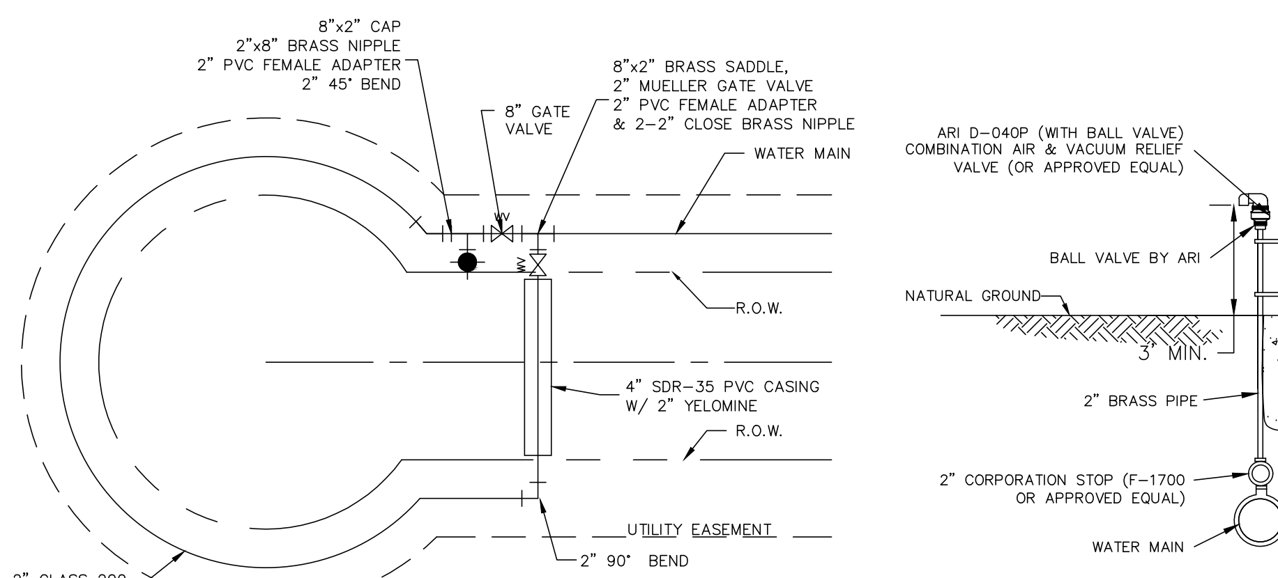
AIR RELEASE VALVE N.T.S.
